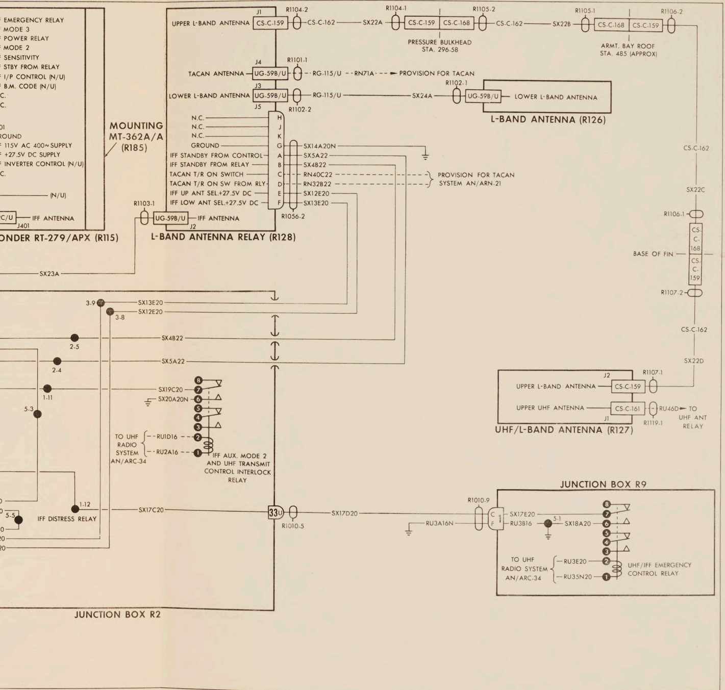
FIG. 4 IFF AN/APX-6A
