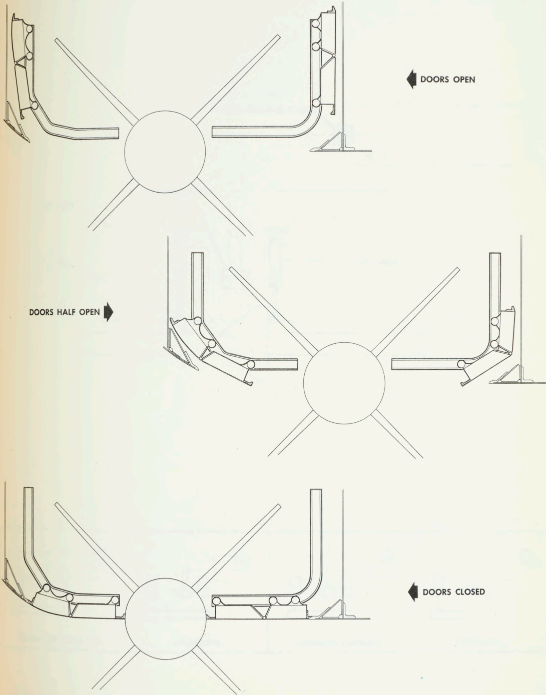
FIG. 6 MISSILE FIN DOORS
